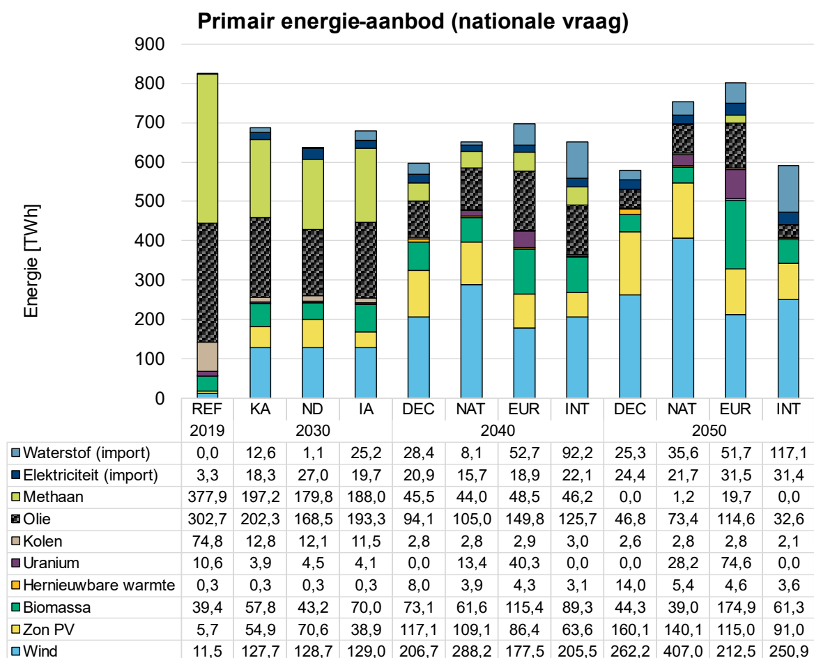
Figuur 7. Primair energieaanbod voor binnenlandse behoefte, inclusief grondstoffen en syngas. De benodigde biomassa voor de productie van SAF is niet gemodelleerd in het ETM en niet opgenomen in deze figuur. Vanaf 2030 bestaat een deel van het aanbod olie uit geïmporteerde pyrolyse-olie. Zie ook sectie 5.2.3.
